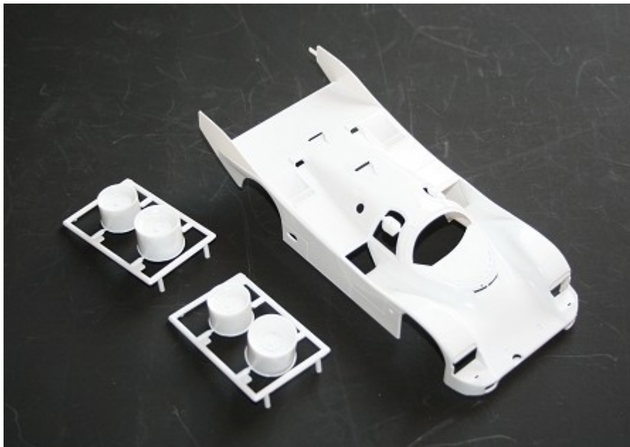
Einteilige Karosserie und Radnaben
