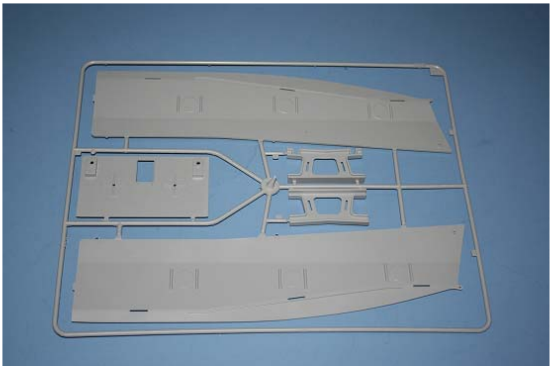
Innenseitenteile mit Bootsständer
