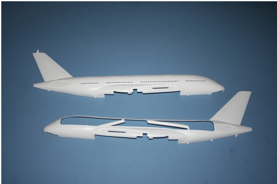
Rumpfteile mit aufgeschnittener linken Rumpfhälfte
